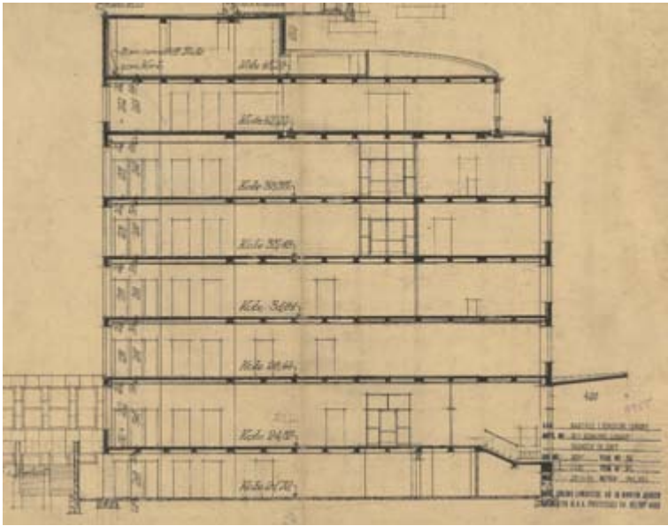
Bygningsnit fra opførelsen.
